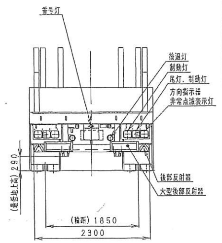
東邦TE47H4C3S型 セミトレーラ外観四面図
